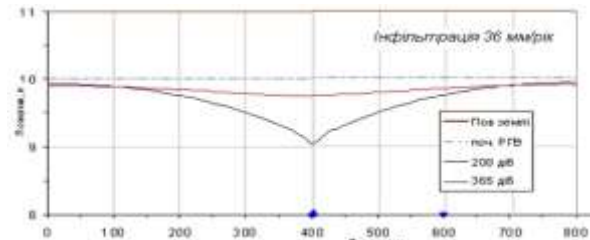
Рисунок 3. Вигляд депресійної кривої при роботі систематичного горизонтального дренажу (розрахункові параметри)
