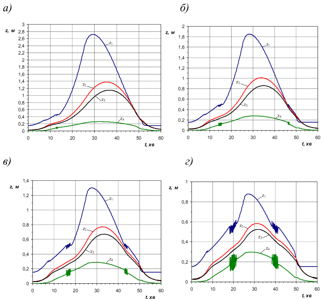
Рисунок 2 – Динаміка зміни рівнів рідини при різних діаметрах байпасного трубопроводу: а) d=150 мм; б) d=180 мм; в) d=210 мм; г) d=250 мм ( q_{20}=100 л/(с·га); n=0,71 ; \psi_{mid}=0,95 ; L/B=5 ; n_1=0,013 ; i_o=0,01 ; Q_r=136,26 л/с; K_{оч}=0,22 ; Q_{ос}=30 л/с)
