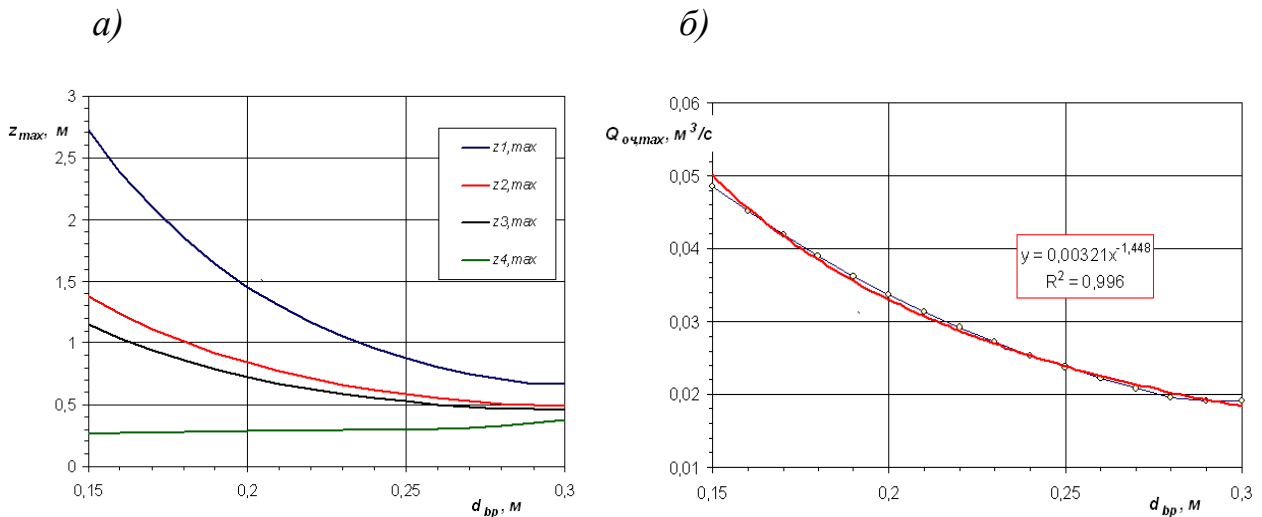
Рисунок 4 – Вплив діаметра d_{bp} на максимальні значення рівнів та витрат: а) залежність максимальних рівнів води в системі; б) залежність максимальної очисної витрати Q_{оч, max} від діаметра d_{bp} (при тих самих умовах, що на рис. 2)
