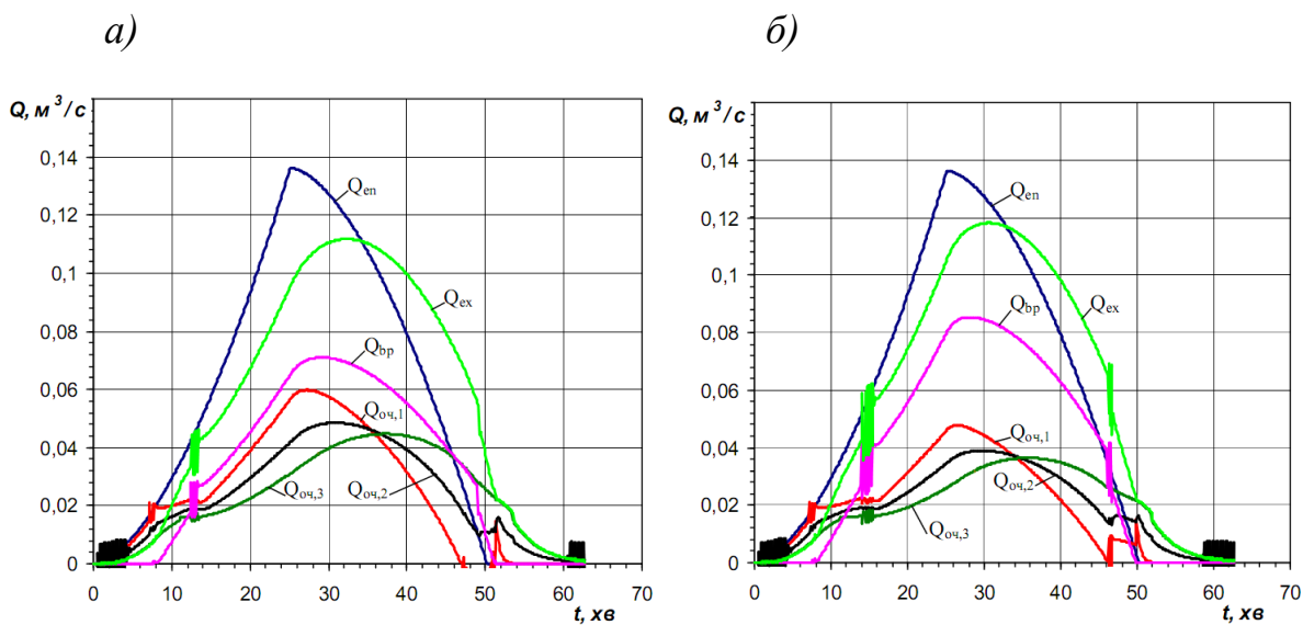
Рисунок 3 – Графіки зміни витрат води в системі при різних діаметрах байпасного трубопроводу для: а) d=150 мм; б) d=180 мм (при тих самих умовах, що на рис. 2)
