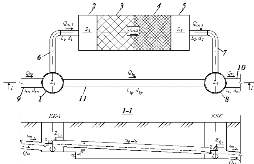
Рисунок 1 – Розрахункова схема блочних ОСДСВ з байпасним трубопроводом:
