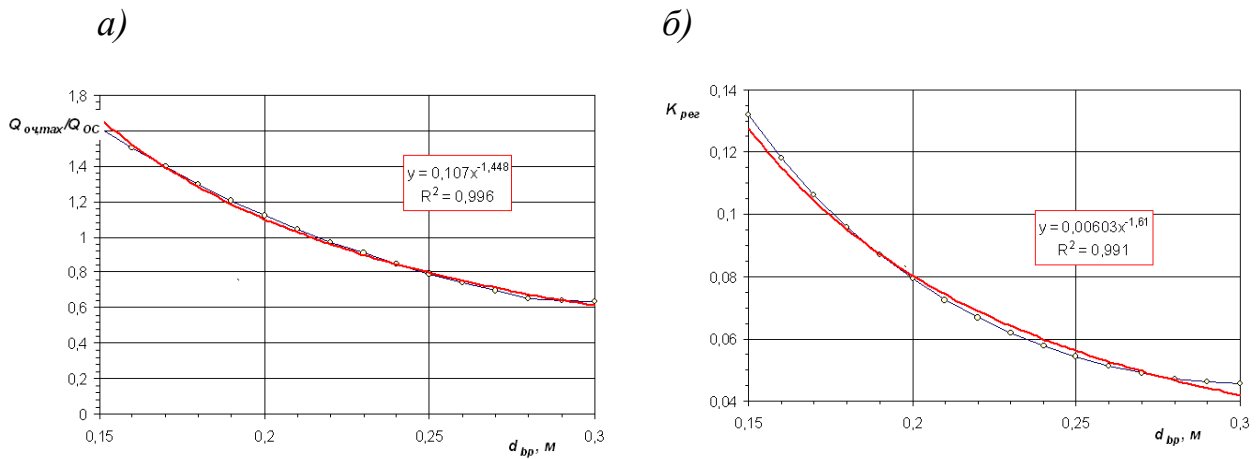
Рисунок 5 – Вплив діаметра байпасного трубопроводу на значення: а – відносної максимальної очисної витрати Q_{оч,max}/Q_{ОС} ; б – коефіцієнта регулювального об'єму ОСДСВ K_{рег} (при тих самих умовах, що на рис. 2)
