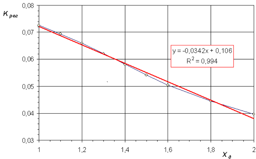
Рисунок 6 – Залежність коефіцієнта регульовального об'єму ОСДСВ K_{рег} від безрозмірної тривалості дощу X_{\partial} ( d_{bp}=210 мм та при тих самих умовах, що на рис. 2)
