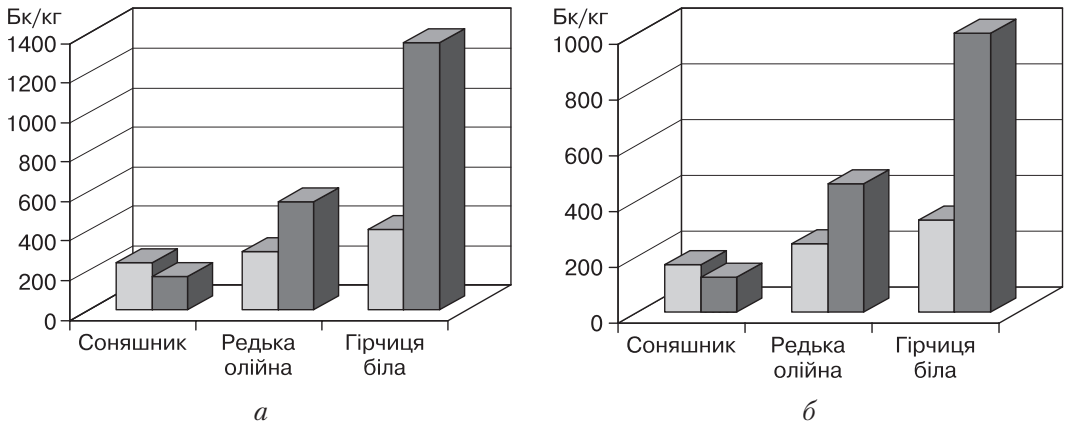
Рис. 2. Питома активність ^{137}\text{Cs} у сільськогосподарських культурах, вирощених в умовах стаціонарного дослідження: а) без добрив; б) з використанням добрив — \text{N}_{30}\text{P}_{60}\text{K}_{90} ; □ — зелена маса; ■ — зерно
