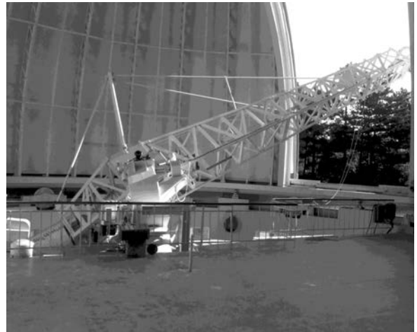
Fig. 1: Coronagraph KG-2.
