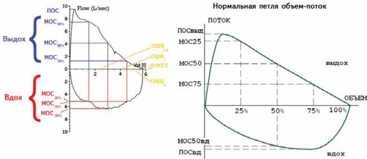
Рис. 1. Примеры расчётных петель "объём-поток".
