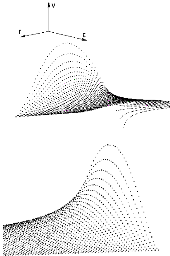
Рис. 1. Зависимость скорости жидкости от радиуса и полярного угла \varepsilon
