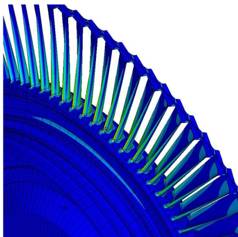
Рис. 7. Напряженное состояние колеса (верные колебания рабочего колеса, 2 узловых диаметра)
