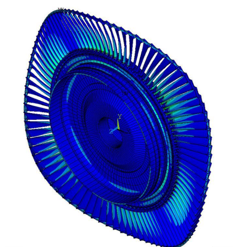
Рис. 6. Напряженное состояние колеса (веерные колебания рабочего колеса, 3 узловых диаметра)
