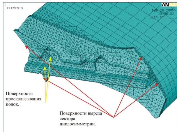
Рис. 2. Бандажная полка. Обеспечение условий циклосимметрии и проскальзывания.
