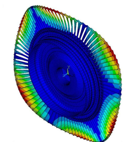
Рис. 5. Преимущественно веерные колебания рабочего колеса, 3 узловых диаметра, f = 274 Гц
