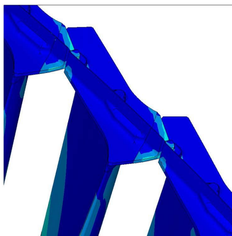
Рис. 8. Напряженное состояние в полке в случае разрезной связи (верные колебания, 2 узловых диаметра)
