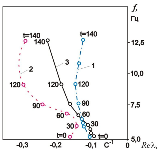
Рис. 1. Годографы доминирующего собственного значения матрицы системы для различных решений задачи (1) параметрической оптимизации демпфера
