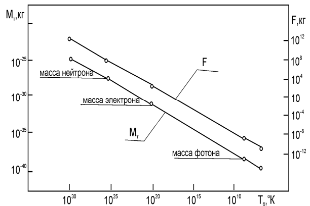
Рис. 5. Влияние температуры барионного кванта ( T_b ) на изменение усилия взаимодействия в би-веществе (при P_b = 101325,52 Па)
