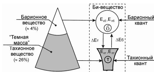
Рис. 1. Модель взаимодействия барионного (б) и тахионного (т) квантов: E_{пб}, E_{пт} – кинетическая и потенциальная энергии квантов; \Delta E_{б, т} – работы, затрачиваемые на взаимодействие
