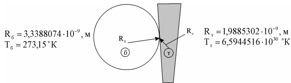
Рис. 6. Соотношение температур барионного и тахионного квантов в их пограничной области при P_b = 1011325,52 \text{ Па}
