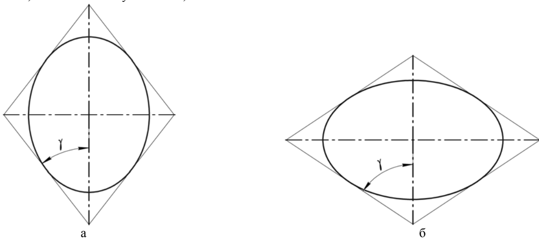
Рис. 4. Эквивалентное зерно:
