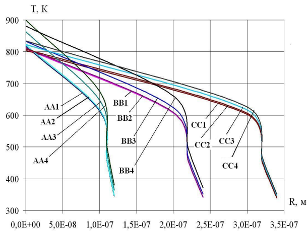
Рис. 4. Распределение температуры, полученной в результате воздействия каплей AA i , BB i и CC i (i=1,4), по радиусам действия температур подложки железа в различных плоскостях (i=1 – плоскость, расположена на глубине x = 0,5L C ; i=2 – плоскость, расположена на глубине x = 0,5L A ; i=3 – плоскость, расположена на глубине x = 0,5L B ; i=4 – плоскость, расположенная на глубине x = 0,8L B )
