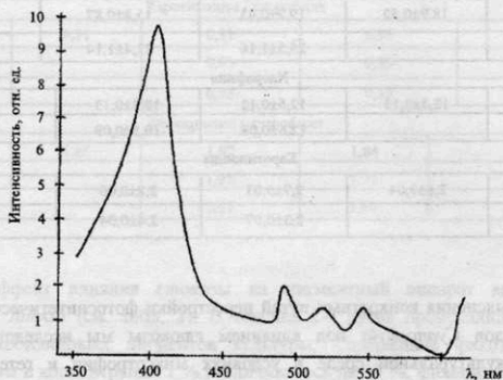
Рис. 3. Спектр возбуждения флуоресценции культуральной среды N. linckia (Roth) Born. et Flah. (1 %-я глюкоза, \lambda_{\text{фильтр}} = 618 нм)
