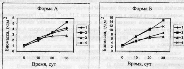
Рис. 2. Динамика накопления биомассы лауренции форм А и Б в опытах, проведенных по плану табл. 2.
