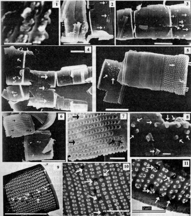
Рис. 5. Тонкое строение створки Aulacoseira islandica (O. Müller) Simonsen из оз. Ханка (1, 5-11) и р. Амур (2-4). 1 – велум; 2 – расположение двугубых выростов вблизи кольцевидной диафрагмы и на удалении от нее; 3-4 – вариабельность локализации двугубых выростов на створках разных клеток одной колонии (белые стрелки), кольцевидная диафрагма (черные короткие стрелки); 5 – расположение двугубых выростов группой в центре загиба створки (тонкие стрелки), на загибе створки видна ступенька (широкая стрелка); 6 – двугубые выросты на внутренней стороне загиба створки (белые стрелки), наружные отверстия двугубых выростов (черные стрелки); 7 – фрагмент створки 6; 8 – двугубые выросты, ориентированные в разные стороны; 9 – расположение двугубых выростов продольными рядами; 10 – фрагмент створки 9; 10, 11 – каналы двугубых выростов связаны своим основанием с ареолами. Масштаб 1, 8 – 1 мкм; 10, 11 – 2 мкм; 7 – 2,5 мкм; 2-6, 9 – 10 мкм. СЭМ (1-8), ТЭМ (9-11).
