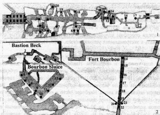
Рис. 1. Схема пунктов отбора проб в казематах Люксембурга: 1 – галерея Бок (1-20 – номера отобранных проб), 2 – галерея Петрусс (22 – номера отобранных проб).
