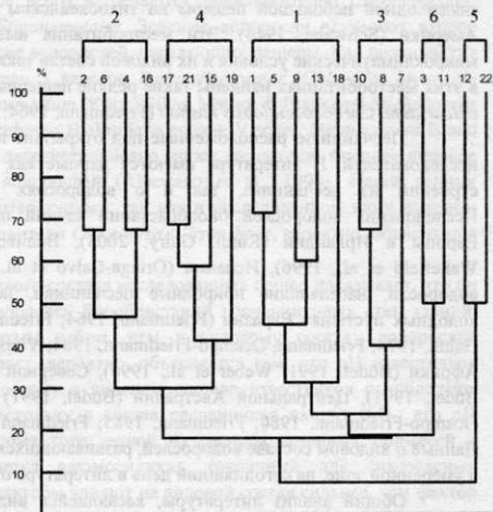
Дендрограмма 2. Основные альгогруппировки галерей Петрус: 1-6 – альгогруппировки, 1-22 – номера исследованных проб.
