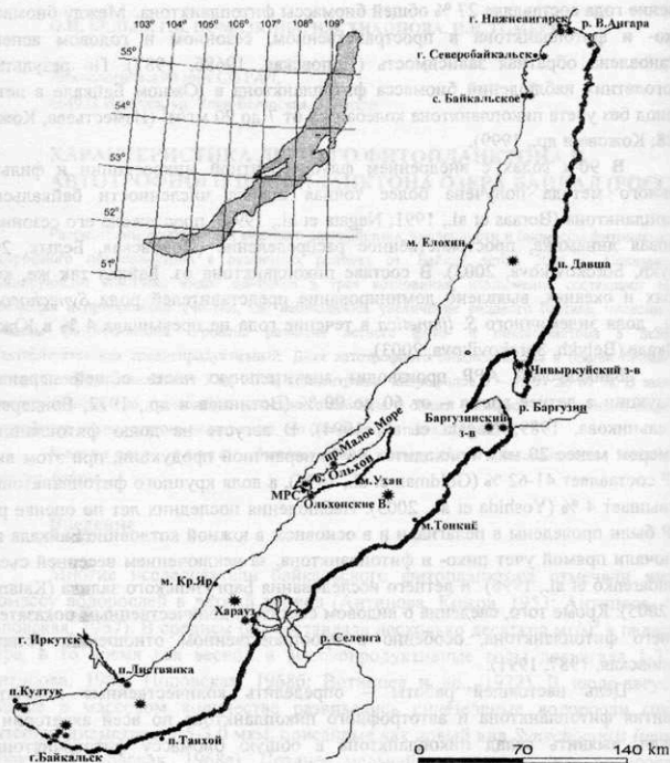
Рис. 1. Схема расположения станций отбора проб в августе 2005 г. на оз. Байкал.
