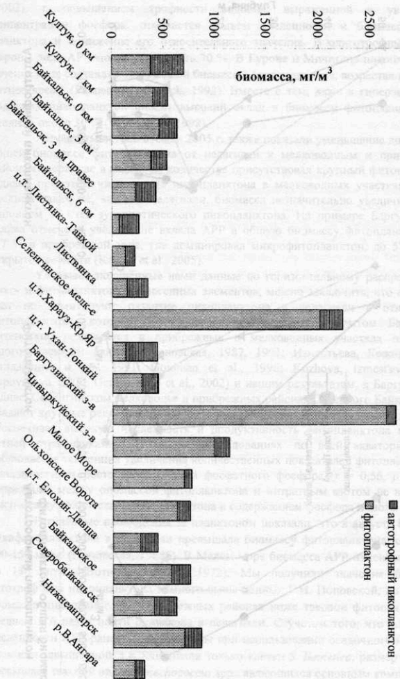
Рис. 5. Горизонтальное распределение биомассы автотрофного пикопланктона и фитопланктона по всей акватории оз. Байкал.
