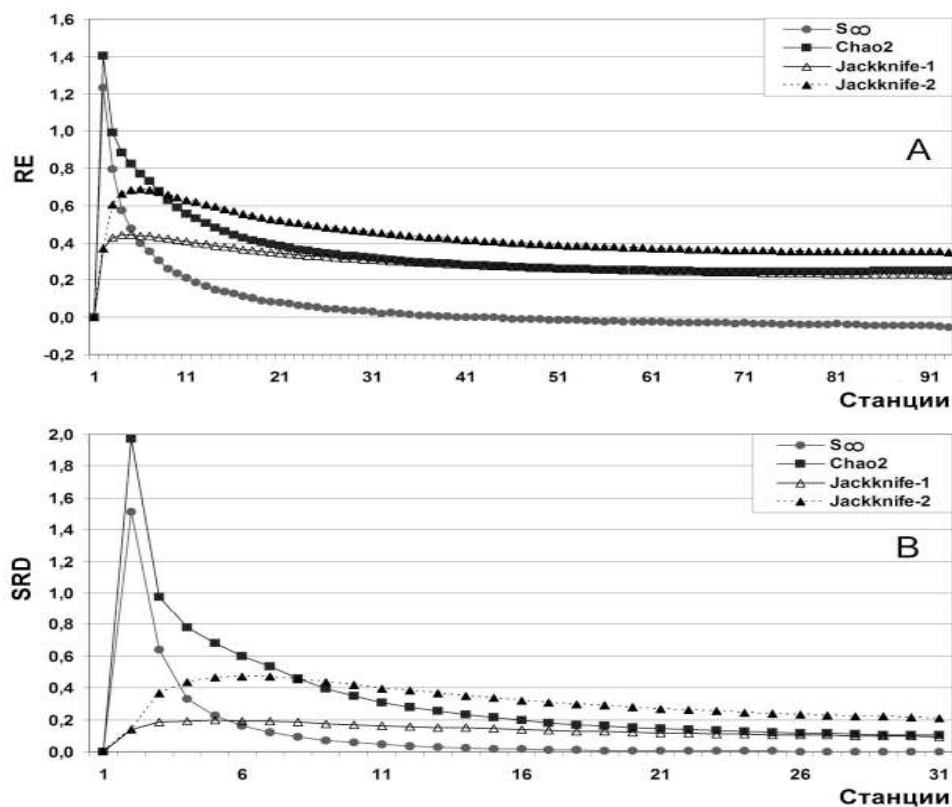
Рис. 8. Оценка погрешности значений эstimаторов ( S_{\infty} , Chao-2, JN-1 и JN-2) на основе показателей относительной ошибки (RE) (A) и квадратичного отклонения (SRD) (B). На графике RE приведены данные для всех 93 проб, а на графике SRD – для первых 30 проб (для большей наглядности)
