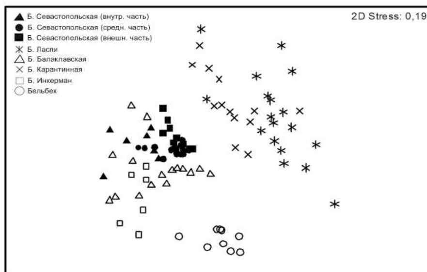
Рис. 2. Результаты MDS-ординации 93 станций (по трансформированной в степени 0,25 матрице сходства численности диатомовых)
