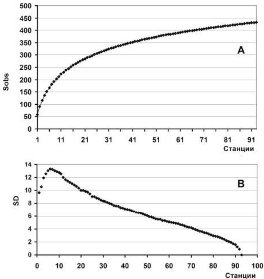
Рис. 7. Кривые накопления числа видов диатомовых ( S_{obs} ), фактически встреченных у побережья ЮЗ Крыма (A), и изменения величины стандартного отклонения (SD) среднеожидаемого числа выявленных видов (B), рассчитанные с учетом рандомизации для возрастающего ряда числа проб
