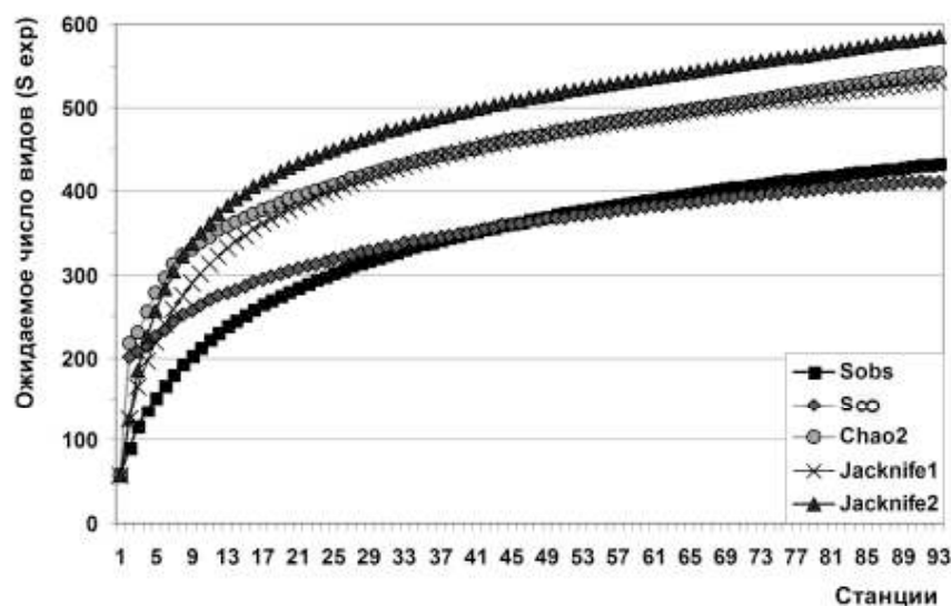
Рис. 6. Кумулятивные кривые ожидаемого числа видов диатомовых ( S_{exp} ) для ЮЗ Крыма, построенные с учетом рандомизации всех 93 проб для фактического найденного в пробах числа видов ( S_{obs} ), а также на основе расчетов 4 эстиматоров ( S_{\infty} ; Chao-2; Jack-knife-1 и Jack-knife-2)
