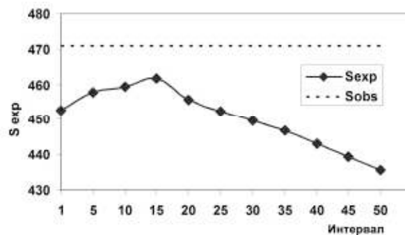
Рис. 9. Изменение ожидаемого числа видов диатомовых ( S_{exp} ), рассчитанного с учетом разной ширины интервала между парами последовательно взятых проб при построении линейных регрессий S_{obs}(n) = f(S_{obs}(n+1)) на основе эстиматора S_{\infty} . На графике для сравнения показано пунктиром общее число фактически выявленных видов ( S_{obs} = 471 )
