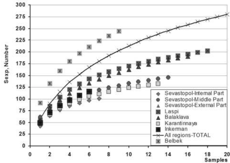
Рис. 3. Кумулятивные кривые расчетно-ожидаемого прироста числа видов S_{exp} (по методу рандомизации) для отдельных полигонов ЮЗ Крыма с разным количеством станций (от 7 до 18) и усредненная кривая, построенная для возрастающей последовательности с учетом всех полигонов (93 станции)
