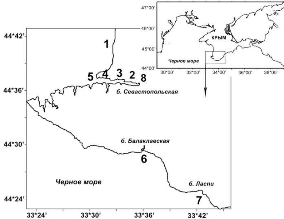
Рис. 1. Карта-схема отбора проб диатомовых водорослей бентоса на полигонах вдоль побережья ЮЗ Крыма. 1 – Бельбек; 2–4 – участки б. Севастопольской (2 – внутренняя, 3 – средняя, 4 – внешняя); 5 – б. Карантинная; 6 – б. Балаклавская; 7 – б. Ласпи; 8 – Инкерман
