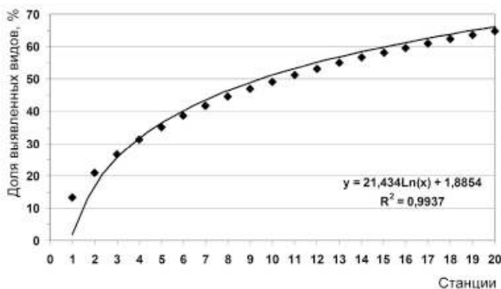
Рис. 4. Доля выявленных видов (в % от 433 видов) в зависимости от числа проб. Параметры уравнения рассчитаны для всех полигонов (93 станции)
