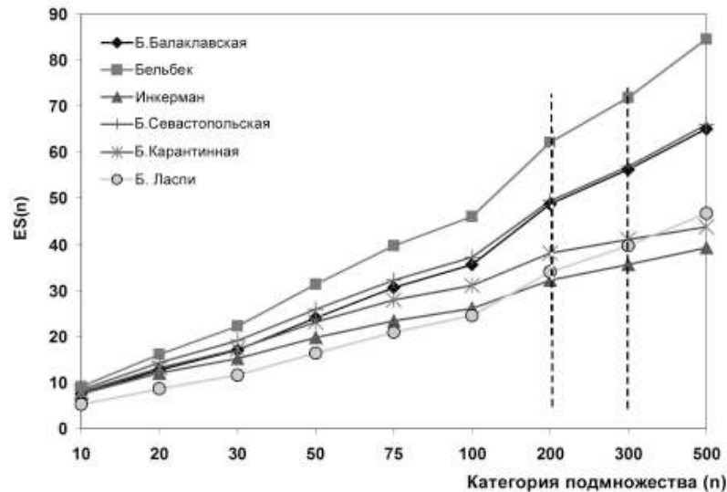
Рис. 5. Изменение ожидаемого числа видов ES(n) для разных полигонов ЮЗ Крыма в зависимости от размера условных подмножеств, состоящих из разного числа особей ( n )
