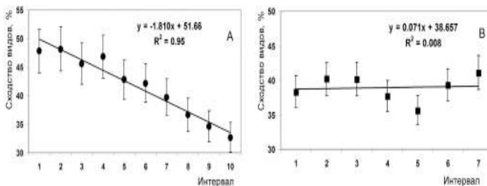
Рис. 10. Тренды в изменении среднего видового сходства ( AvSim \pm SD ) для комбинаций попарно взятых проб при разной ширине интервала между их исходной последовательностью (A – б. Балаклавская, B – б. Карантинная)
