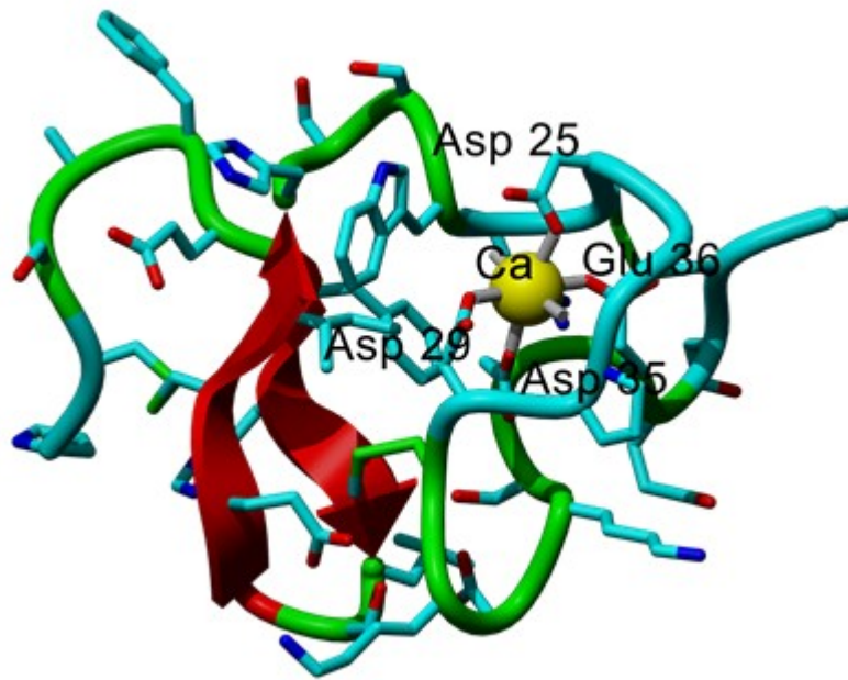
Рис. 10. Структура CR5 модуля LDLR человека [56] (PDB код 1AJJ).
