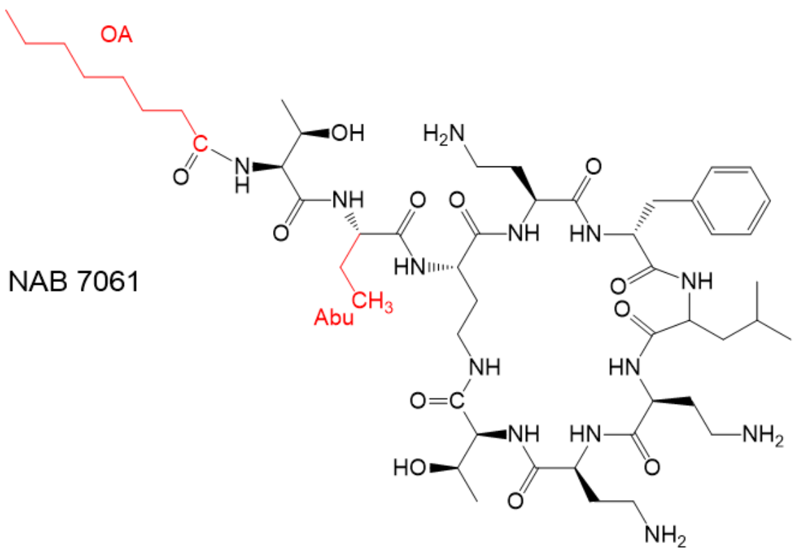
Рис. 5. Химическая структура производного полимиксина Ser3-PmB(3-10).
