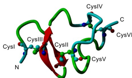
Рис. 15. Характерная трехмерная организация CR повторов. Цистеиновые остатки, образующие дисульфидные связи, показаны с помощью шаро-стержневой модели.
