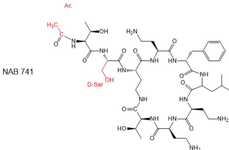
Рис. 8. Химическая структура производного полимиксина NAB 741
