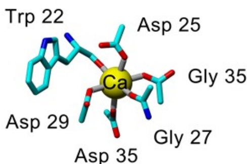
Рис. 14. Ион Ca^{2+} и координированные им отрицательно заряженные аминокислотные остатки и карбонильные группы остова CR5 домена LDLR человека [56].
