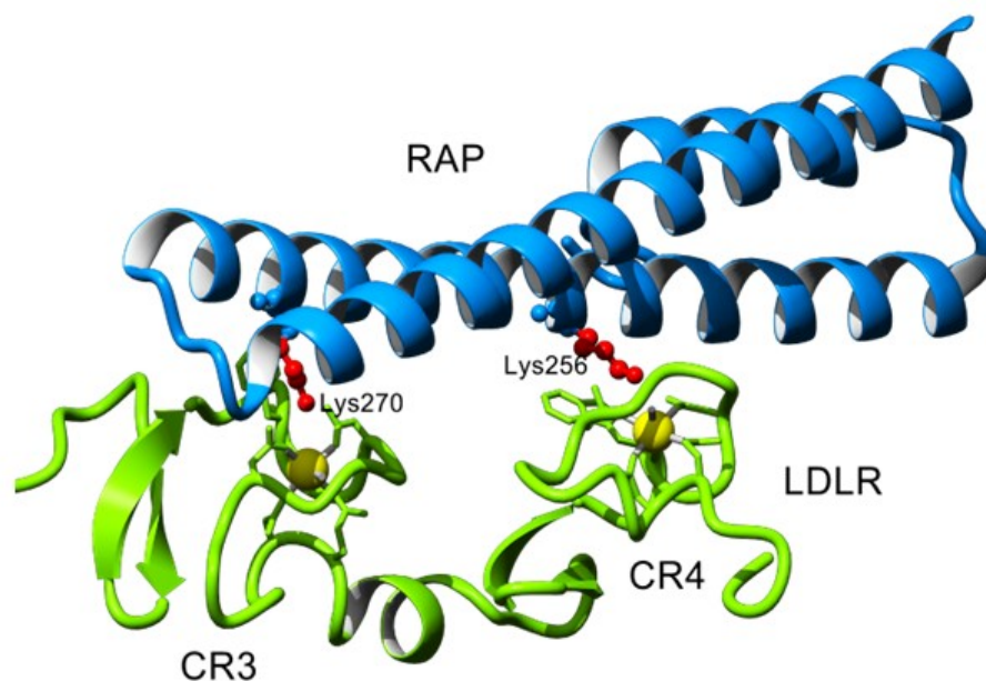
Рис. 18. Структура комплекса RAP протеина с LDL-рецептором [75]. Катионные остатки лизина выделены красным цветом. Атомы водорода не показаны.
