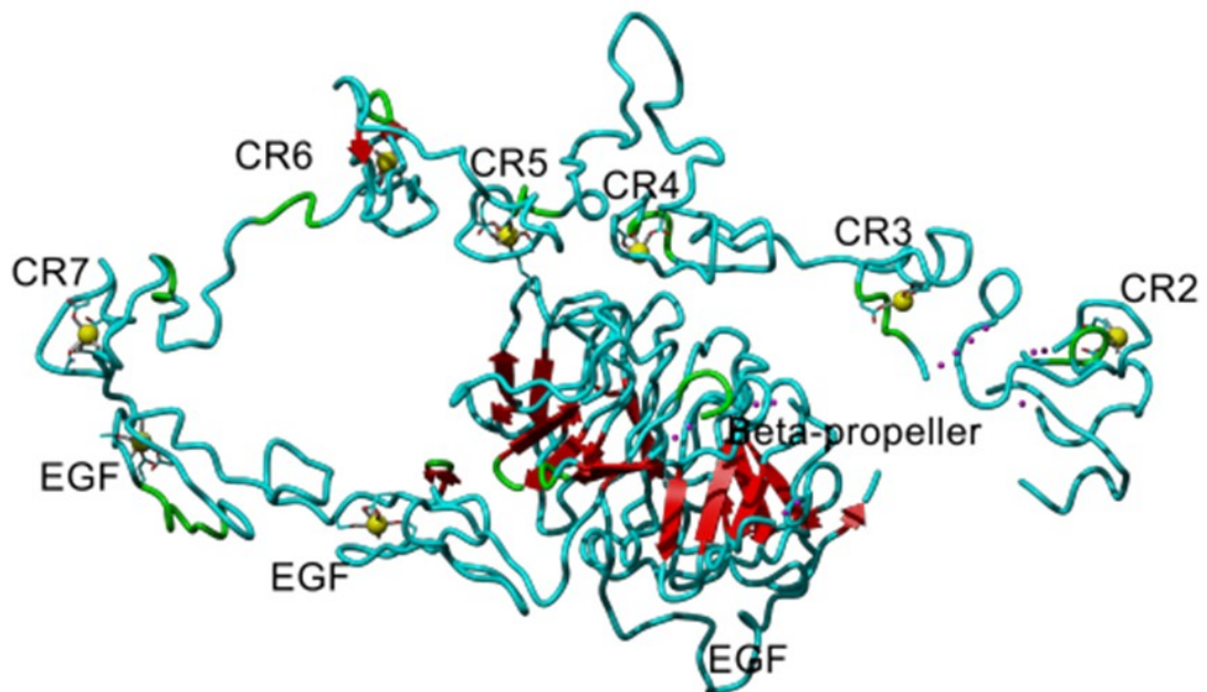
Рис. 13. Структурные модули LDLR человека [59] (PDB код 1N7D)
