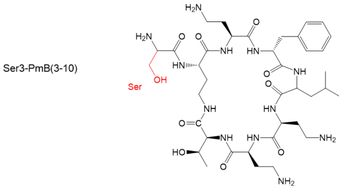
Рис. 5. Химическая структура производного полимиксина Ser3-PmB(3-10).
