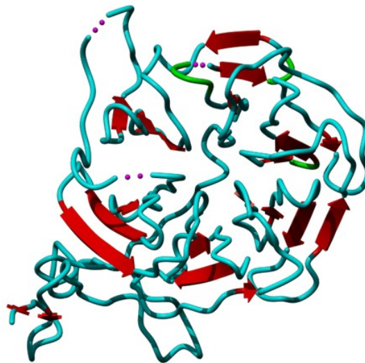
Рис. 12. Структура \beta -пропеллерного домена LDLR человека [58] (PDB код 1HJQ).
