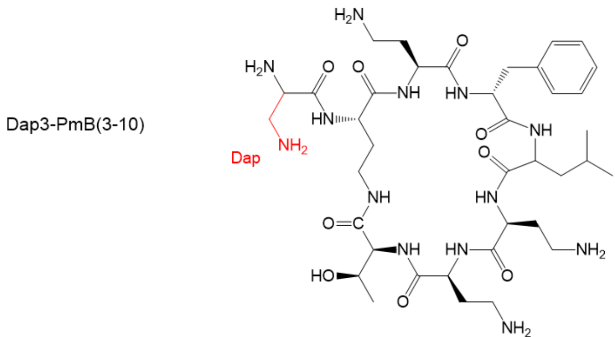
Рис. 4. Химическая структура производного полимиксина Dap3-PmB(3-10).
