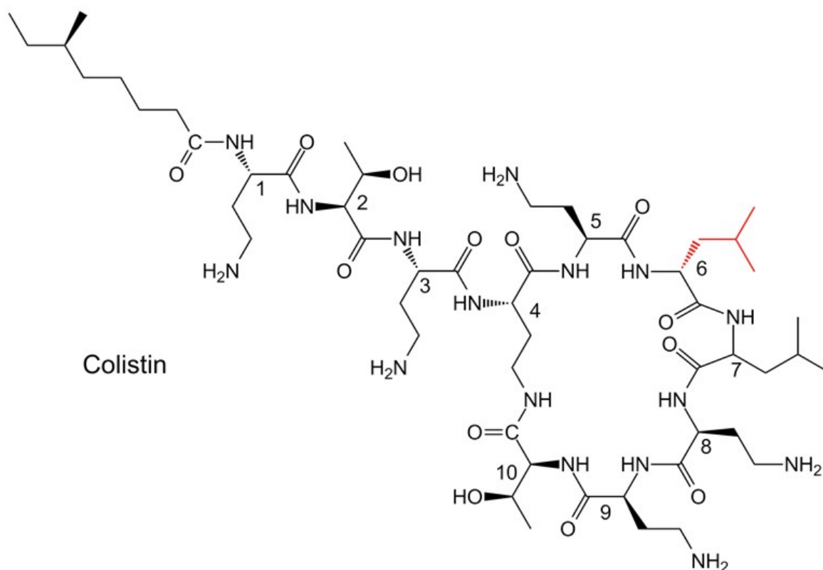
Рис. 2. Химическая структура колистина (полимиксина E 1 ). Отличия от структуры полимиксина В 1 выделены красным цветом.
