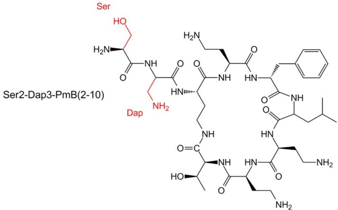
Рис. 3. Химическая структура производного полимиксина Ser2-Dap3-PmB(2-10).
