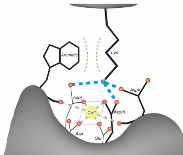
Рис. 17. Универсальный механизм связывания катионных лигандов лиганд-связывающими повторами рецепторов LDLR-семейства [75]. Положительно заряженный атом азота лизинового остатка (Lys) катионного лиганда выделен синим цветом, атомы кислорода кислотных остатков (Asp, Glu) лиганд-связывающих повторов – красным, а связанный кальций в лиганд-связывающем повторе – желтым цветом.
