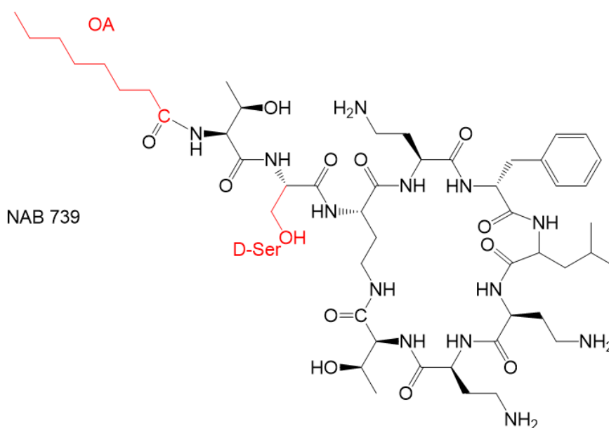
Рис. 7. Химическая структура производного полимиксина NAB 739
