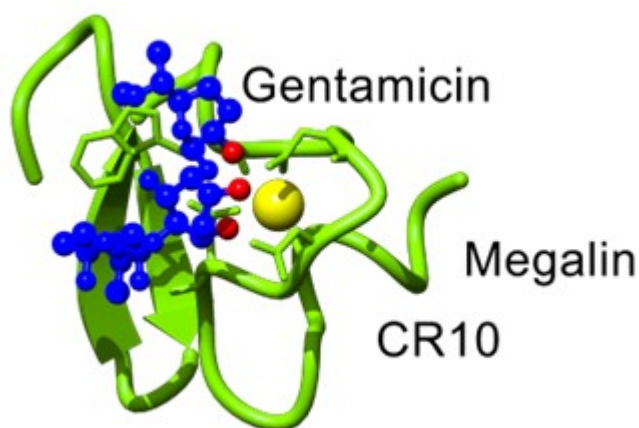
Рис. 19. Структура комплекса гентамицина с лиганд-связывающим доменом CR10 мегалина человека. Гентамицин выделен синим цветом, а его катионные аминогруппы – красным цветом. Атомы водорода не показаны.
