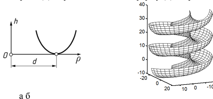
а б Рис. 2. Схема утворення поверхні за заданою кривою осевого перерізу: а) розташування кривої в плоскій системі координат; б) поверхня, утворена гвинтовим рухом заданої кривої
