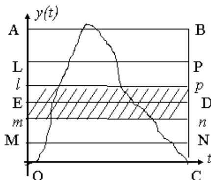
Рис. 1. Зона неопределённости срабатывания реального ИИ
