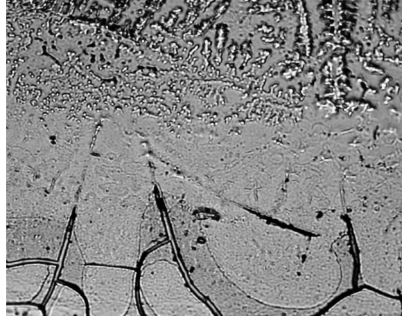
Рис. 2. Дрібні точкові вкраплення аморфної та проміжної зони у вигляді кристалів та хаотичні тріщини периферичного поясу. Збільшення (1:100).
