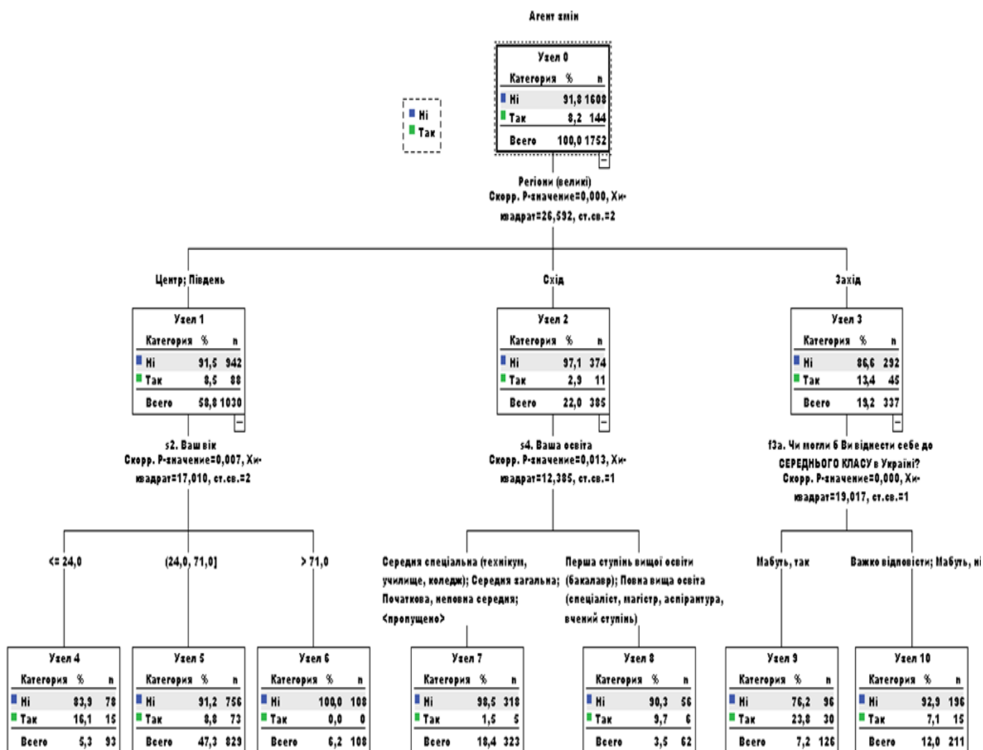
Рисунок 2 - Класифікаційне дерево
