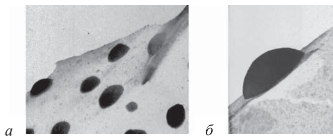
Рис. 3. Электронно-микроскопическое изображение островкового конденсата ( а , \times 20\,000 ) и отдельного островка висмута ( б , \times 40\,000 ) на наклонных участках пленки германия
