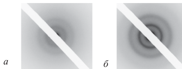
Рис. 2. Микродифракция пленок германия непосредственно после препарирования (а) и после отжига при температуре 610 К в течение 15 ч (б)
