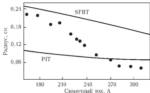
Рис. 3. Зависимость размеров оторвавшихся капель от величины силы тока при сварке стальной проволокой диаметром 1,2 мм в смеси Ag + 2 % O 2 . Сравнение экспериментальных (точки) данных с расчетными (сплошные линии), полученными с помощью методов SFBT и PIT [22]
