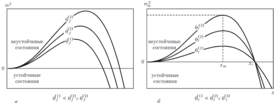
Рис. 5. Влияние силы тока (а) и поверхностного натяжения (б) на скорость распространения неустойчивости
