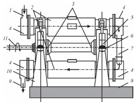
Рис. 2. Схема вибрационной мельницы PALLA-U фирмы KHD HUMBOLDT WEDAG: 1 — загрузочный патрубок; 2 — трубные мельничные камеры; 3 — узлы дебалансных вибровозбудителей; 4 — сменные торцевые днища мельничных камер; 5 — трубные связи; 6 — амортизаторы; 7 — переточный рукав; 8 — виброизолированный фундамент; 9 — выпускной штуцер; 10 — неподвижная рама; 11 — приводной вал
