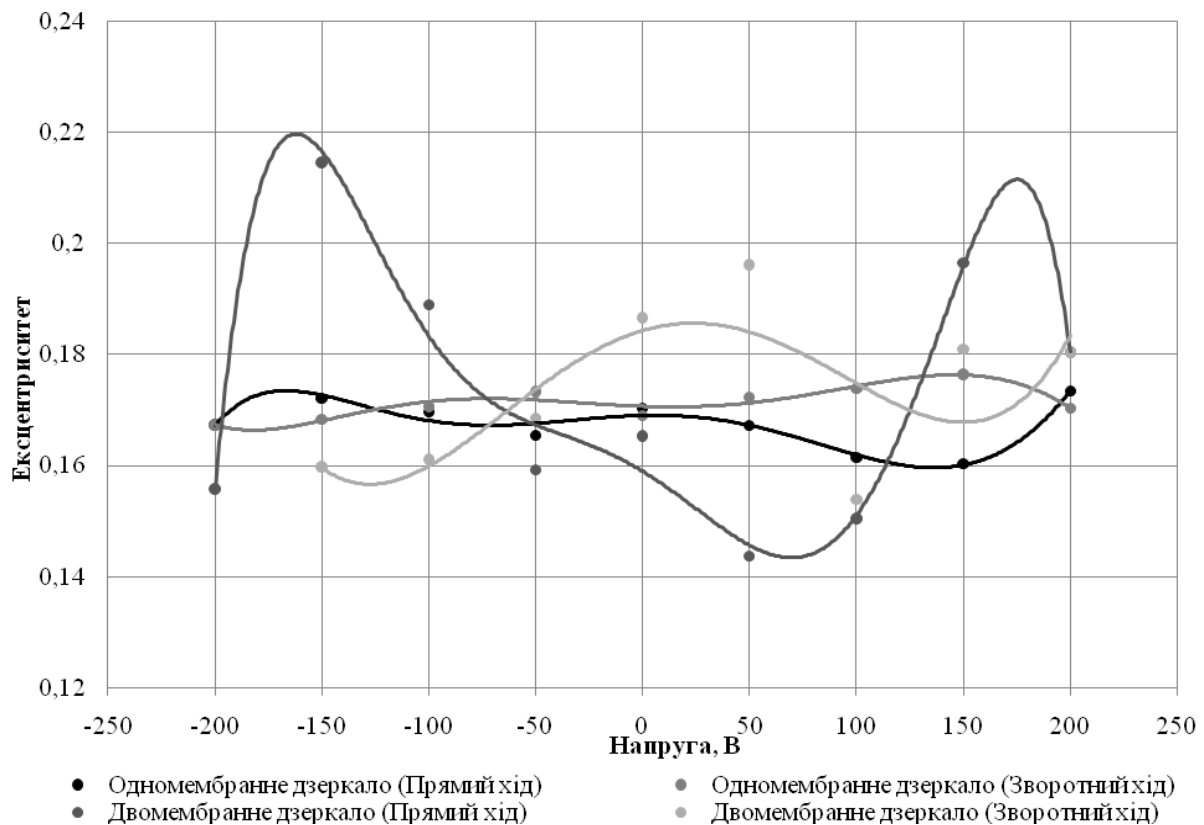
Рис. 9. – Порівняльний графік залежності ексцентриситету поверхні дзеркала обох типів конструкції від напруги
