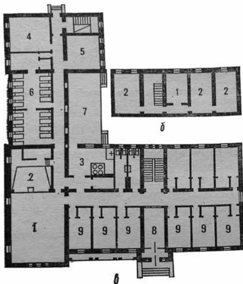
Рис. 2. Проект колективного житла для комуні, 1925 р. (фасад та план будівлі). Автор: Д. Дяченко. 1 – їдальня, 2 – сцена, 3 – кухня, 4 – група для дітей, 5 – клас, 6 – дитяча спальня, 7 – веранда, 8 – сіни, 9 – житлова кімната [5]
