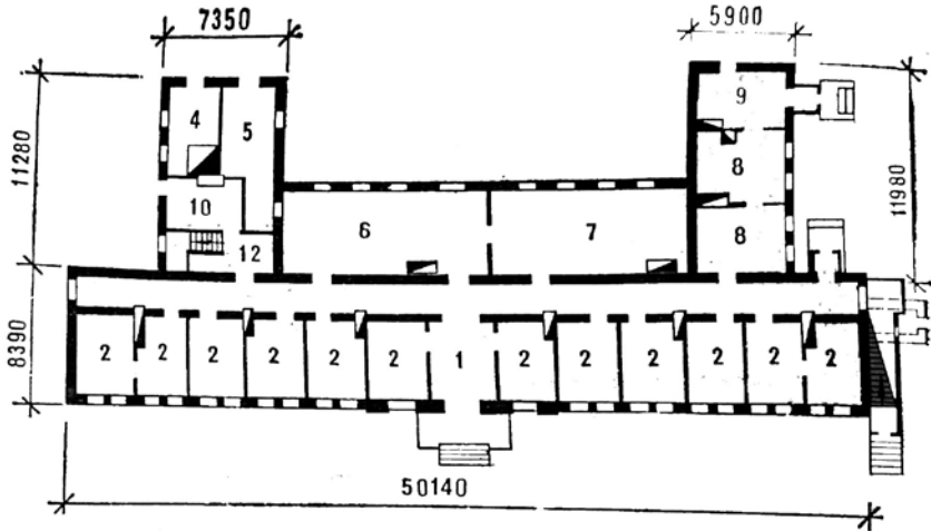
Рис. 3. Житловий будинок у комуні «Здобуток Жовтня» (обміри Ю. Хохла).
