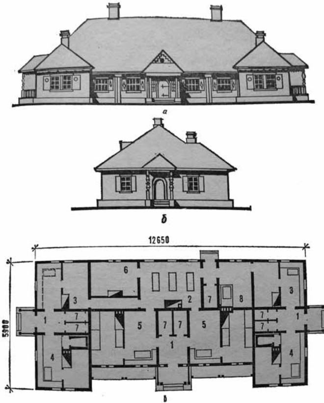
Рис. 1. Проект колективного житлового будинку комуни 1923 р. (фасади та план будинку). Автор: Д. Дяченко. 1 – сіни, 2 – їдальня, 3 – приміщення для сім'ї з 3 чол., 4 – те саме для 4-х, 5 – для п'яти, 6 – приміщення для парубків, 7 – кімрка, 8 – пекарня [5]
