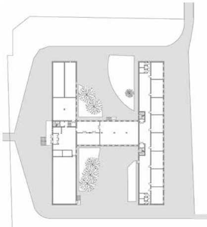
Рис. 1. План першого поверху середньої загально-ноо-світньої школи №50 в м.Києві. Існуючий стан.
