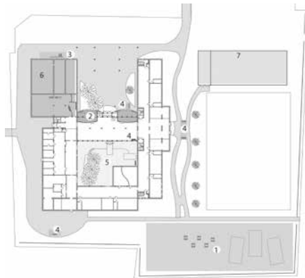
Рис. 2. Проект реконструкції школи.
