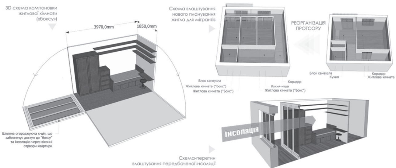
Рис.3 Схема влаштування житла для мігрантів за допомогою житлових «боксів»
