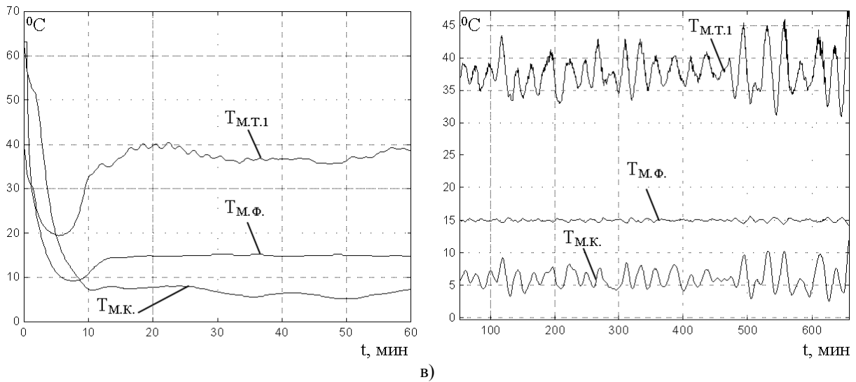
Рис. 2 – Иллюстрация процессов стабилизации температурных режимов в переходных и установившихся процессах для некоторых альтернативных вариантов САУ: а) вариант 1; б) вариант 3; в) вариант 5
