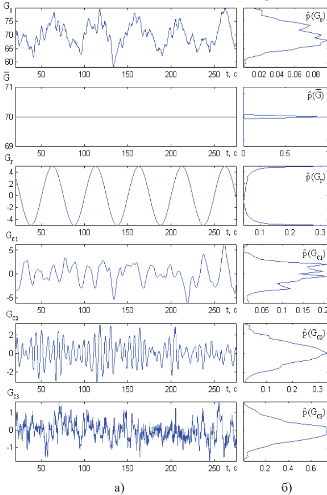
Рис. 2 – Фрагмент реалізації тестової моделі процесу витікання G_0(t) дозуемого матеріалу на стрічку КВДБД та його складових: а) часові діаграми; б) оцінка щільностей імовірності
