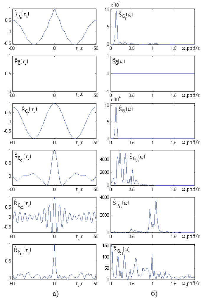
Рис. 3 – Оцінки автокореляційних функцій (а) та спектральних щільностей (б) змінної G_0 та її складових (відповідно до рис. 2)
