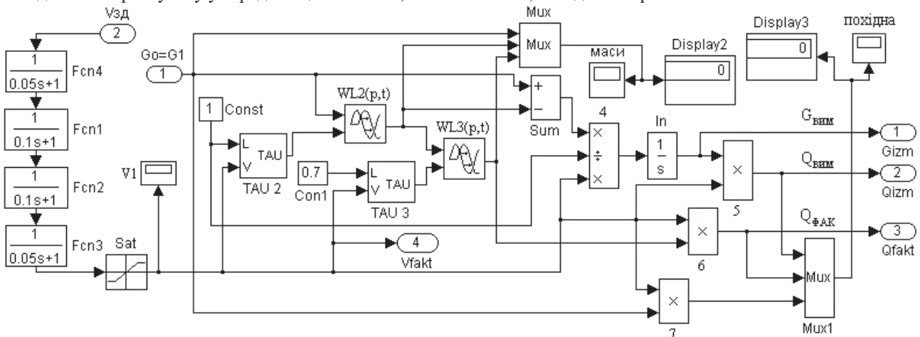
Рис. 6 – Схема моделювання переміщення матеріалу стрічкою конвеєра, його накопичення ваговимірювальною ділянкою, руху стрічки від електроприводу та обчислення вимірюваних значень маси та продуктивності
