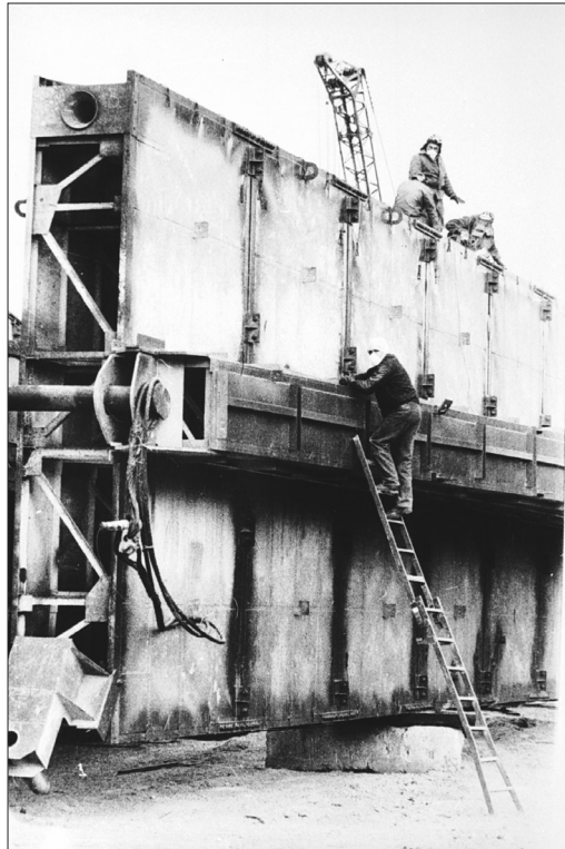
Монтаж металоконструкцій перекриття та бетонування захисної стіни 4-го енергоблоку Чорнобильської АЕС ім. В. І. Леніна. м. Прип'ять Чорнобильського району Київської обл., жовтень 1986 р. ЦДКФФА України ім. Г. С. Пшеничного, од. обл. 0-211130.
