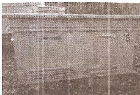
Рис. 2 Вулик з спеціальним пристроєм для органічних кислот, що навішуються над лотком
