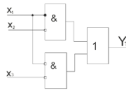
Рис. 4. Функціональна схема функції № 172
