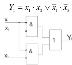
Рис. 2. Функціональна схема функції № 163
