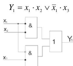
Рис. 1. Функціональна схема функції № 83
