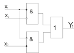
Рис. 3. Функціональна схема функції № 92
