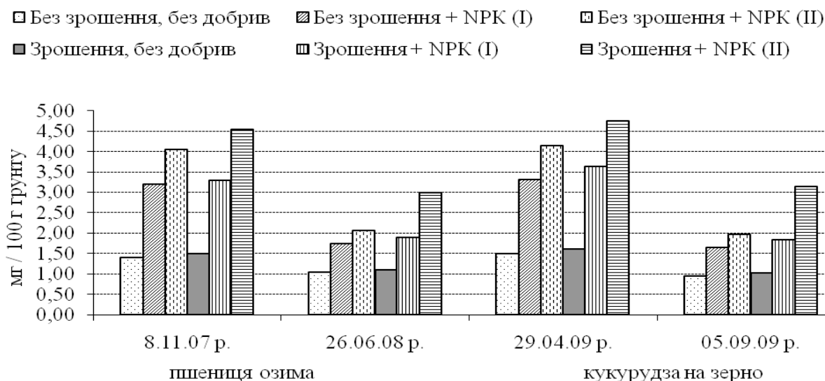
Рис. 3. Динаміка вмісту рухомого фосфору в орному шарі ґрунту залежно від зрошення та мінерального удобрення, мг/100 г ґрунту.
