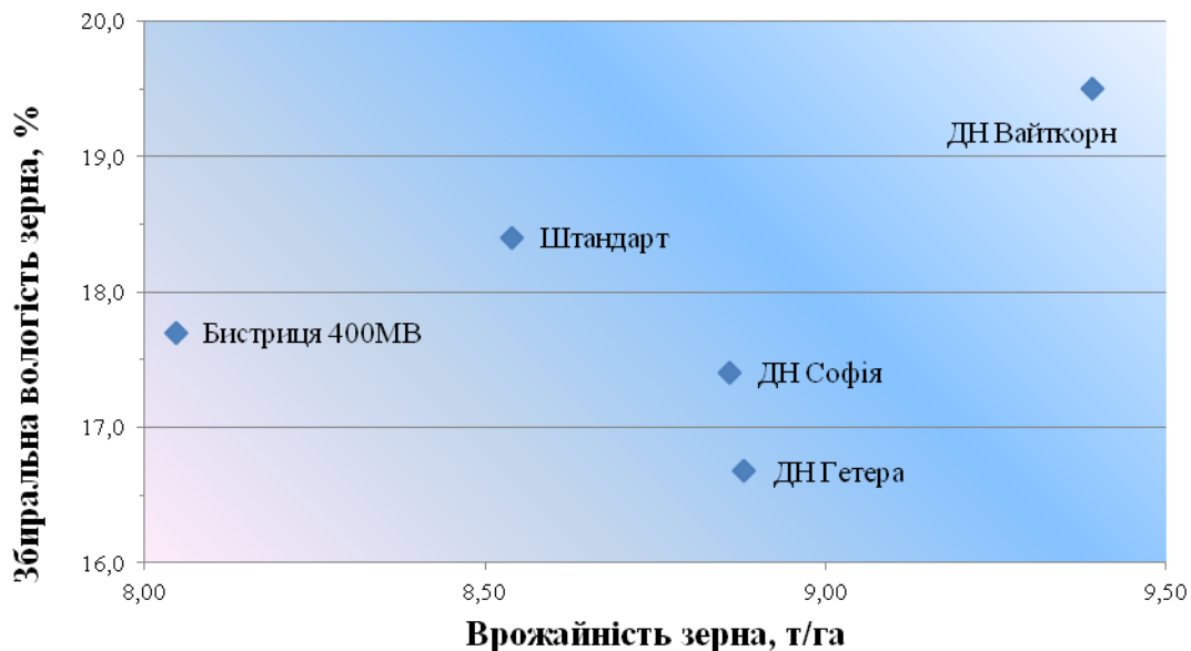
Рис. Найкращі гібриди за співвідношенням урожайності зерна до його збиральної вологості.
