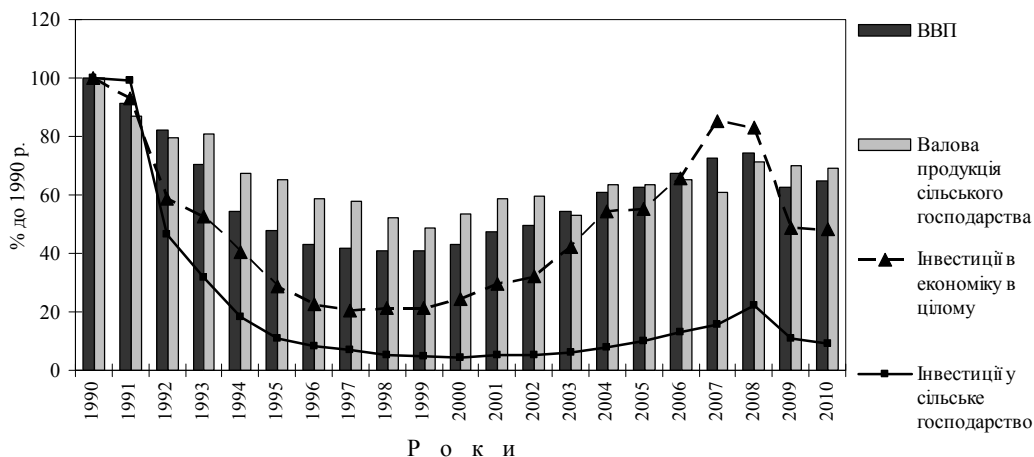
Рис. 1. Динаміка ВВП, виробництва валової продукції сільського господарства та інвестиційних потоків упродовж 1990–2010 рр.
