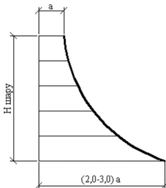
Рисунок 1 - Епюра розподілу в'язучого по висоті захисного шару асфальтобетону, що укладений на мембрану де а - процентна кількість модифікованого бітуму у складі асфальтобетону.
