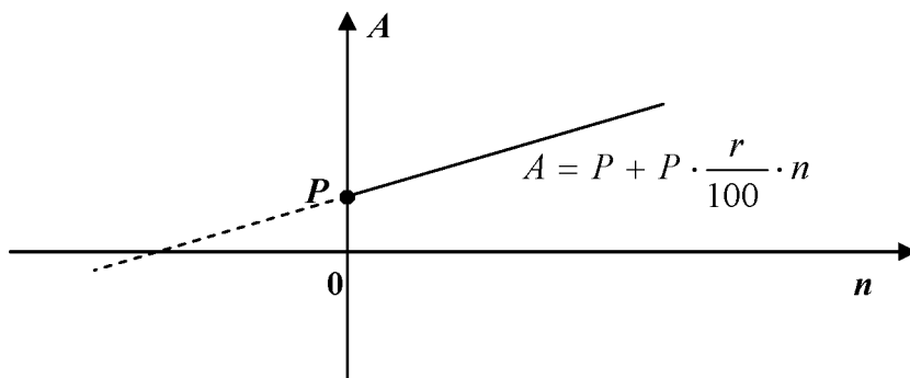
Рис. 1. Графік лінійної функції A = f(n)
