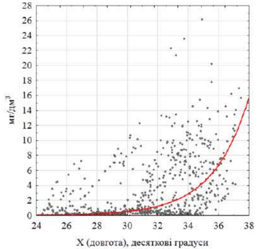
Рис. 3. Просторовий розподіл надходження ґрунтово-ерозійного фосфору до поверхневих вод окремих суббасейнів транскордонного басейну річки Дніпро: а – картограма і модель просторового розподілу, б – південь → північ, в – захід → схід
