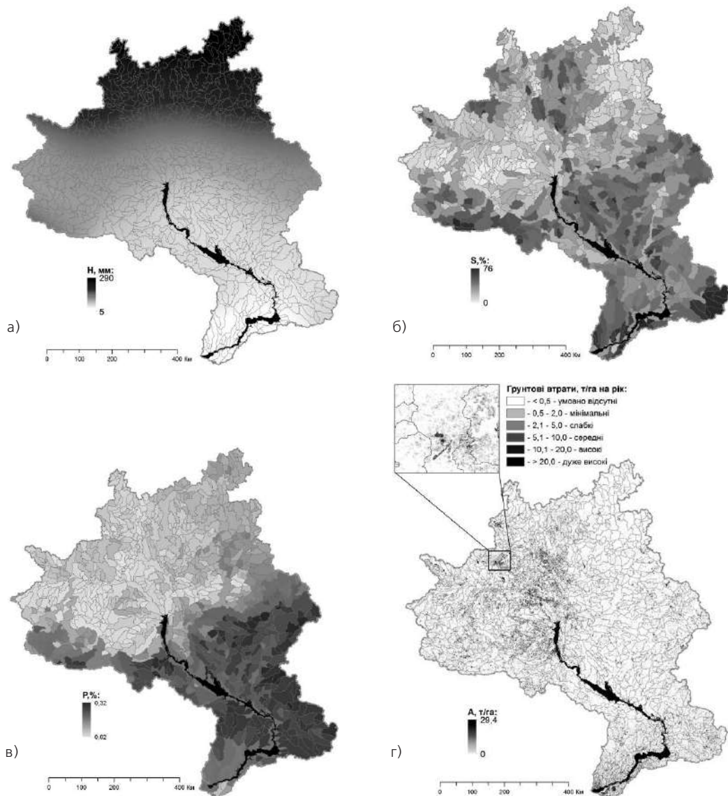
Рис. 2. Розподіл факторів впливу на потенційну небезпеку забруднення фосфором поверхневих вод басейну річки Дніпро: а – середньобагаторічний шар поверхнього стоку води (Н, мм); б – доля ріллі на водозбірній території (S, %); в – вміст валового фосфору в орному шалі (Р, %); г – інтенсивність змиву на пашіні (А, т/га)
