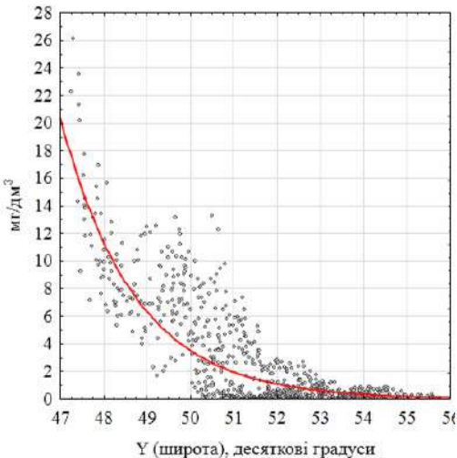
Рис. 3. Просторовий розподіл надходження ґрунтово-ерозійного фосфору до поверхневих вод окремих суббасейнів транскордонного басейну річки Дніпро: а – картограма і модель просторового розподілу, б – південь → північ, в – захід → схід
