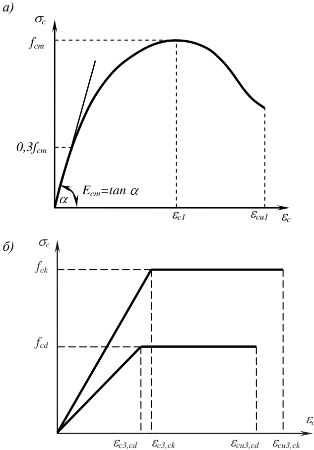
Рис. 1. Діаграма «напруження-деформації» бетону: а) – криволінійна; б) дволінійна
