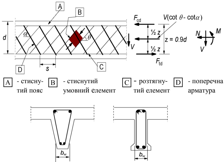
Рис. 4. «Фермова» модель і позначення для елементів з поперечним армуванням
