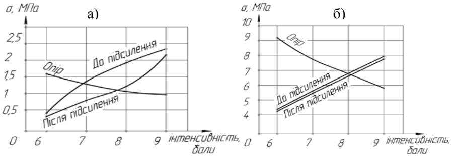
Рис. 3. Опір та максимальні напруження, які виникають в: а) – кам'яній кладці; б) – залізобетонній колоні.
