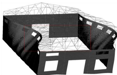
Рис. 2. Деформації споруди при дії сейсмічних навантажень.
