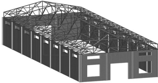
Рис. 1. Просторова модель споруди
