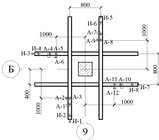
Рис. 4. Схема расстановки тензометров Аистова (А) и индикаторов часового типа (И):
