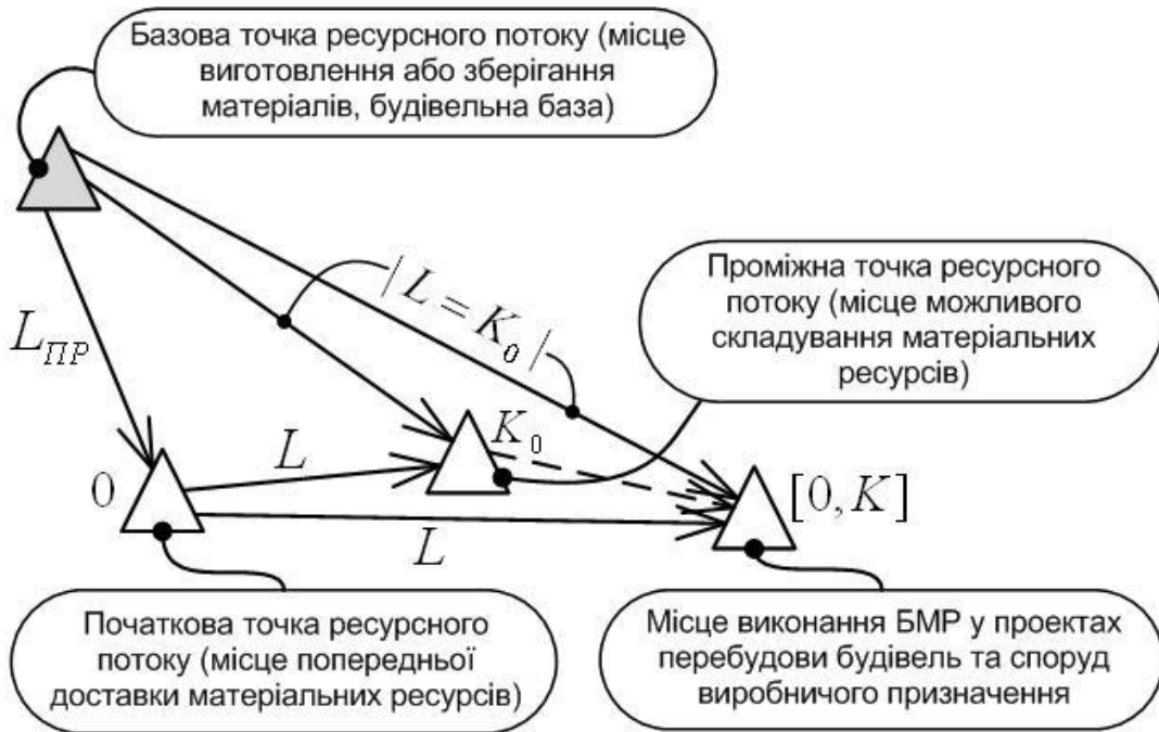
Рис. 2. Узагальнена схема організації системи ресурсного забезпечення проекту із додатковим складом ( L=K_0 )
