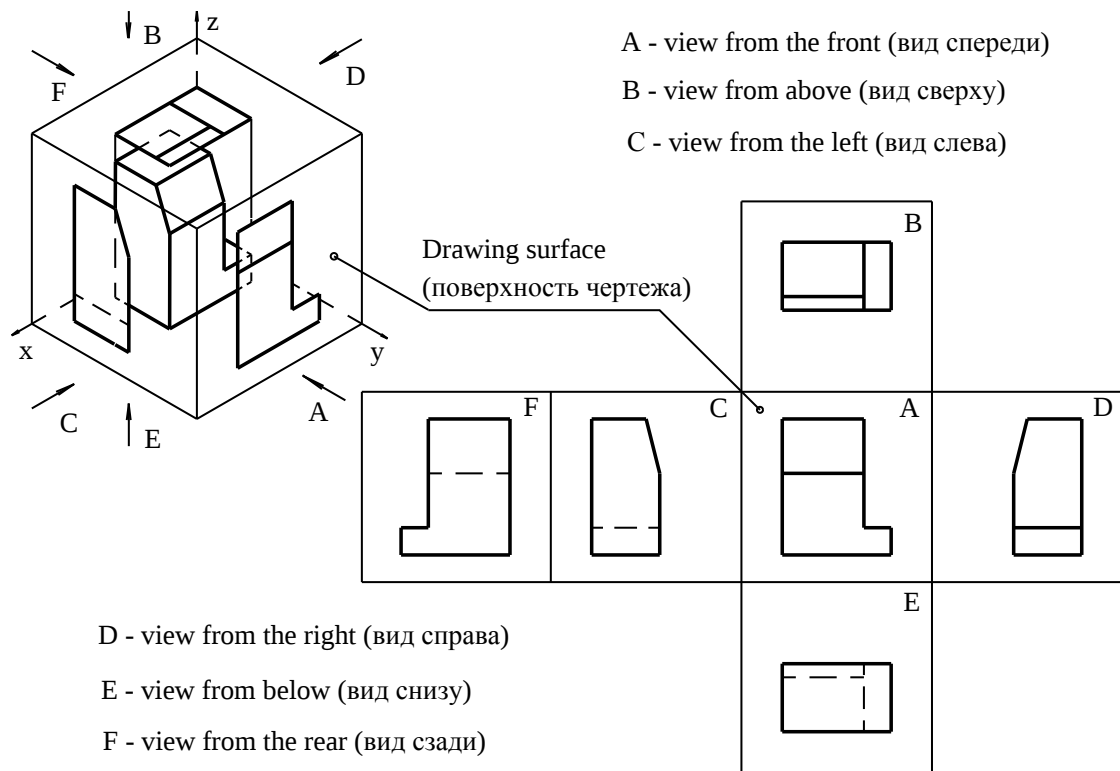
Рис. 2. Стандартное расположение видов изделия для метода третьего октанта
