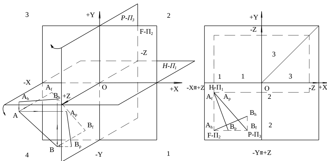
Рис. 4. Комплексный чертеж отрезка прямой линии для третьего октанта в соответствии с международным стандартом
