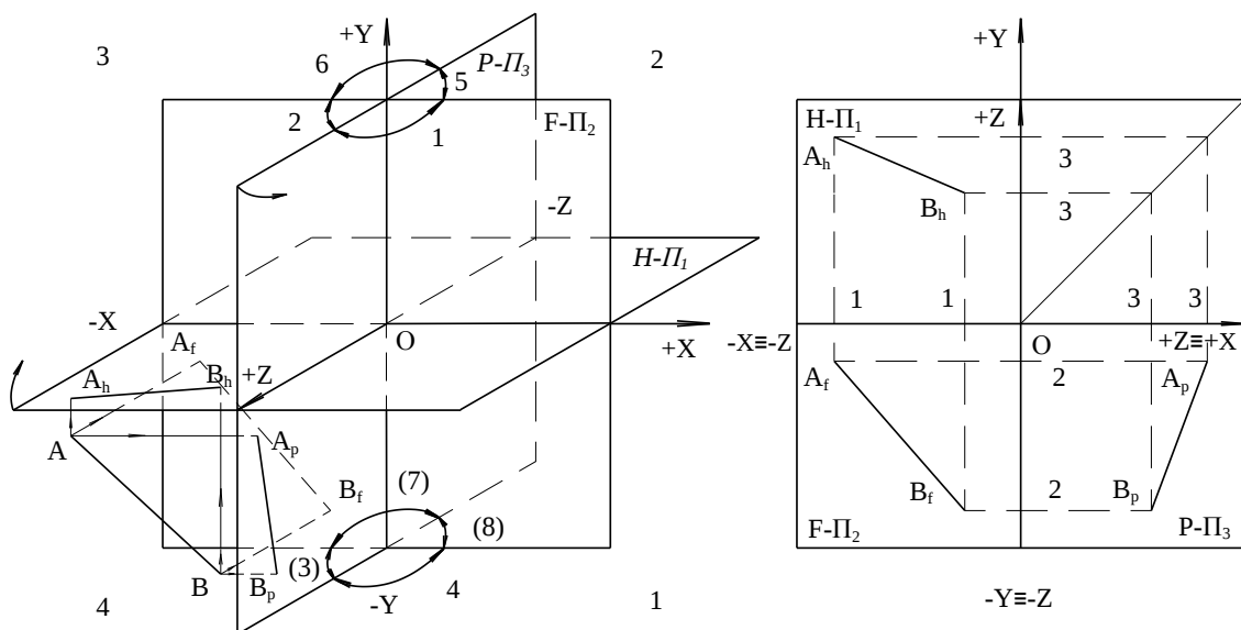
Рис. 3. Комплексный чертеж отрезка прямой линии для третьего октанта в американской системе измерения [11]
