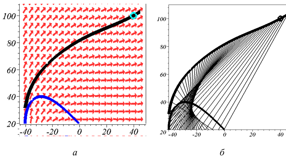
Рис. 6. Поле ізоклін і відбивальна крива ( a ), та сім'я відбитих від неї променів ( б )
