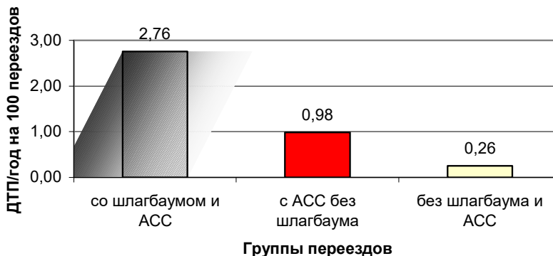
Рисунок 2 - Относительная аварийность на переездах с разным уровнем оборудования
