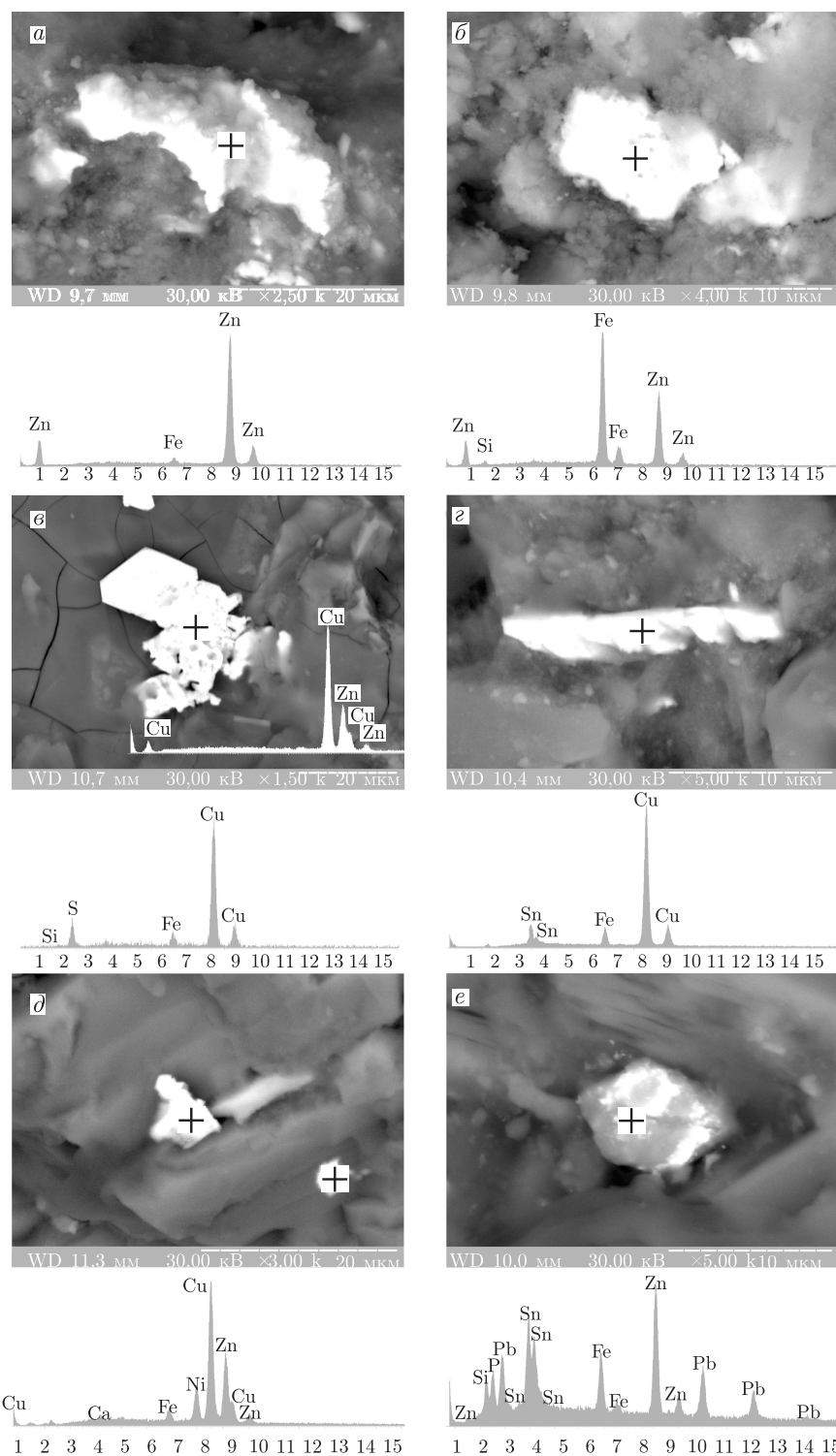
Рис. 3. Самородный цинк с примесью железа (а); цинковое железо (б); цинковая медь (природная латунь) в ассоциации с халькозином (в); железо-оловянная бронза (г); поликомпонентный (Zn–Fe–Ni–Cu) сплав (д); фосфатно-силикатный ксенолит с включениями поликомпонентного (Fe–Sn–Pb–Zn) сплава (е) [а, б — скв. 5514, гл. 272,0 м; в — Малый карьер Иванчи; г, д, е — скв. 5514, гл. 386,0 м]
