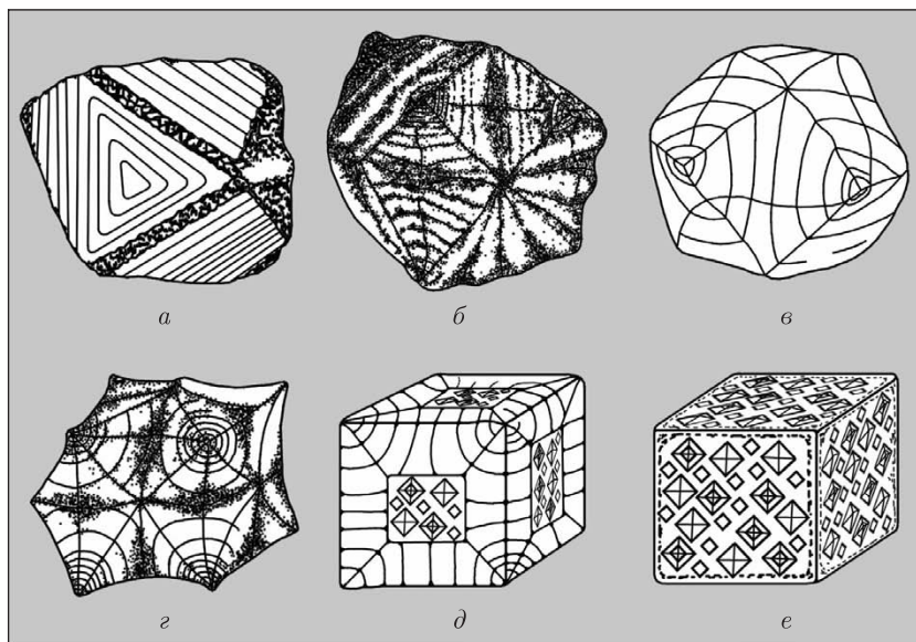
Рис. 3. Зарисовка основних морфологічних типів кристалів зелених мікроалмазів Побужжя–Придністров'я: a — перехідна форма (октаедр-ромбододекаедр); b ; в — різні додекаедроїди; г — тетрагексаедріод; д — комбінаційна форма (куб-додекаедріод); е — куб
