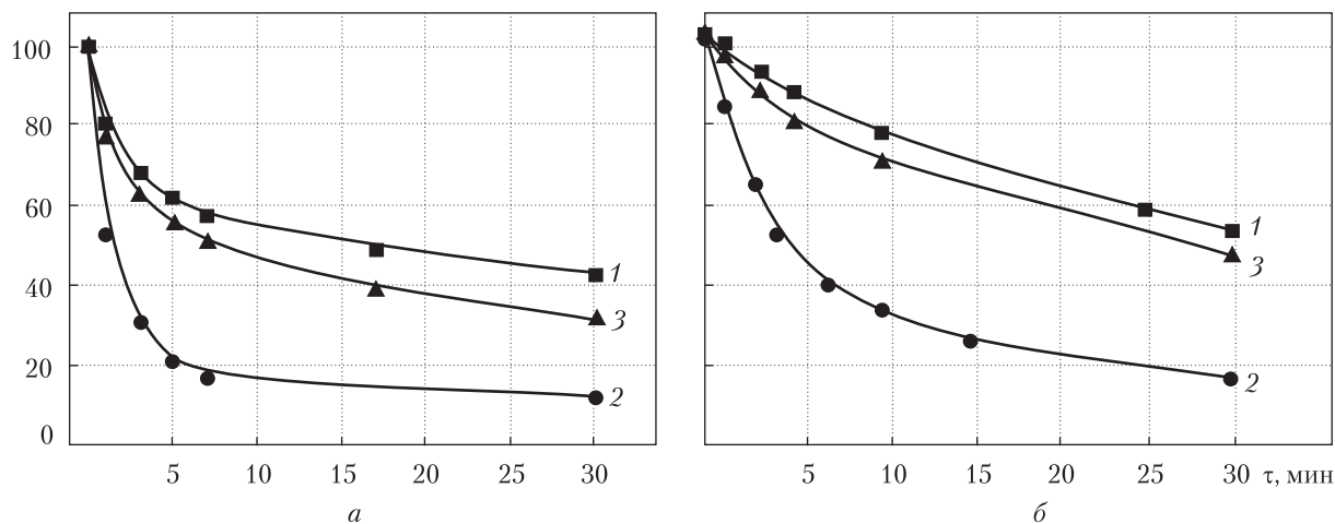
Рис. 1. Кинетические кривые гибели радикала ДФПГ в реакции с экстрактами Vitex cannabifolia (1), Vitex agnus-castus (2), Vitex negundo (3) в стандартных условиях (а) и в среде 0,1 ммоль/л HCl (б). Разбавление исходных экстрактов 1:100. C/C_0 — отношение концентрации радикала в растворе к исходной концентрации, %
